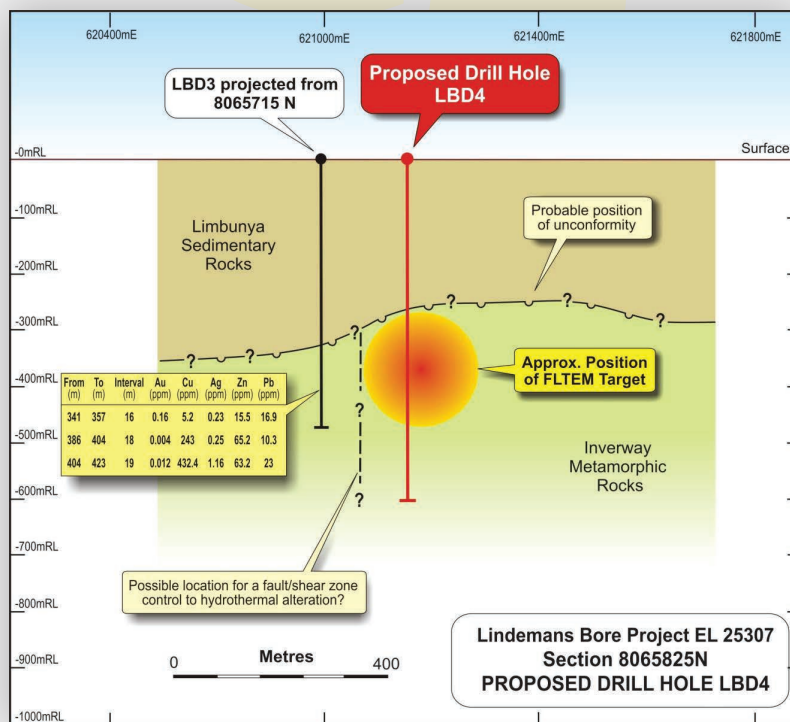
Slika 2 - Predvidena lokacija vrtine LBD4 namerjena v elektromagnetno anomalijo
